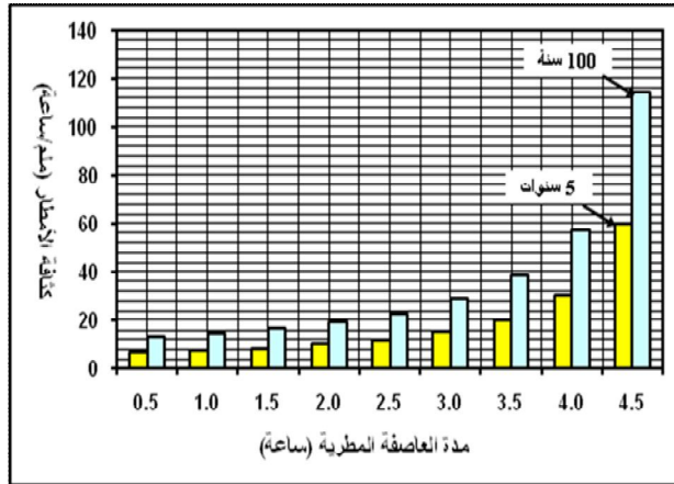
شكل رقم (٨) كثافة الأمطار للعواصف المطرية خلال فترتي الرجوع ٥ و ١٠٠ سنة بمحطة النقرة بنموذج التوزيع الاحتمالي للقيم القصوى (نوع ١)
