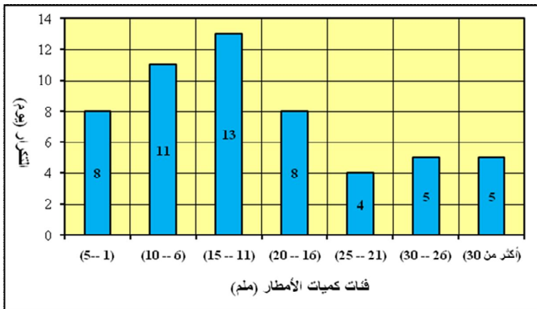
شكل (٣) فئات الأمطار اليومية القصوى المسجلة خلال الفترة ١٩٦٠-٢٠١٦ م بمحطة حائل
