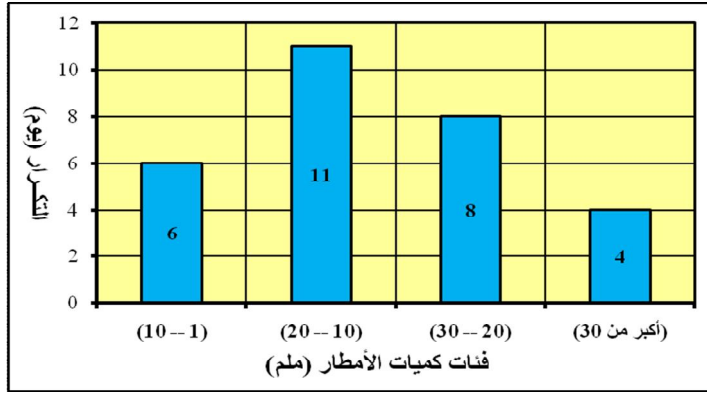
شكل (٥) فئات الأمطار اليومية القصوى المسجلة خلال الفترة ١٩٧١-١٩٩٩ بمحطة النقرة
