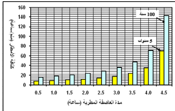
الشكل رقم (١٤) كثافة الأمطار للعواصف المطرية خلال فترتي الرجوع ٥ و ١٠٠ سنة بمحطة الغزالة بنموذج التوزيع الاحتمالي للقيم القصوى (نوع ١)
