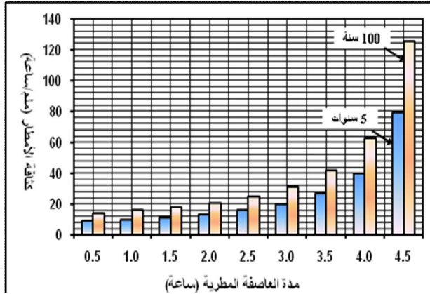
شكل (٩) كثافة الأمطار للعواصف المطرية خلال فترتي الرجوع ٥ و ١٠٠ سنة بمحطة عقلة بن جبرين بنموذج التوزيع الاحتمالي الطبيعي
