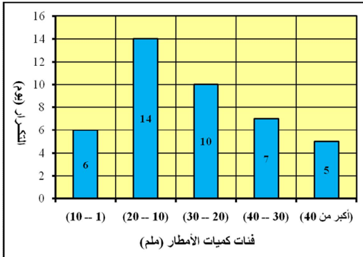
شكل (٦) فئات الأمطار اليومية القصوى المسجلة خلال الفترة ١٩٧٠-٢٠١١ م بمحطة عقلة بن جبرين
