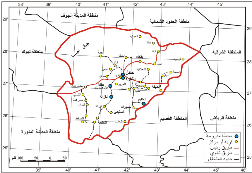
شكل (٢) الموقع الجغرافي للمحطات المطرية بمنطقة الدراسة
