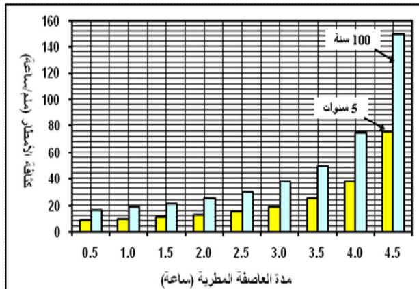
شكل (١٠) كثافة الأمطار للعواصف المطرية خلال فترتي الرجوع ٥ و ١٠٠ سنة بمحطة عقلة بن جبرين بنموذج التوزيع الاحتمالي للقيم القصوى (نوع ١)
