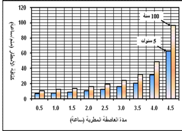
شكل رقم (٧) كثافة الأمطار للعواصف المطرية خلال فترتي الرجوع ٥ و ١٠٠ سنة بمحطة النقرة بنموذج التوزيع الاحتمالي الطبيعي
